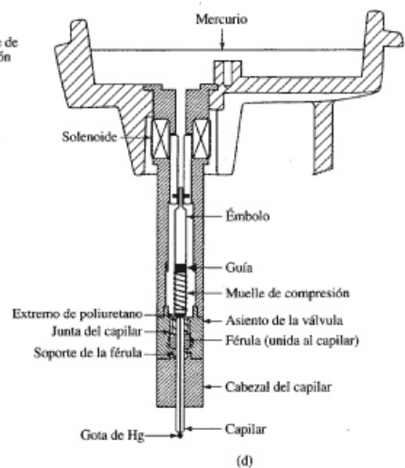
Electrodo de gota estática de Hg
