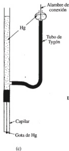
Electrodo de gotas de Hg
