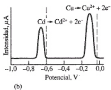
Figura 25-32. (a) Señal de excitación para la determinación por redisolución de \text{Cd}^{2+} y \text{Cu}^{2+} . (b) Voltamperograma de redisolución.
